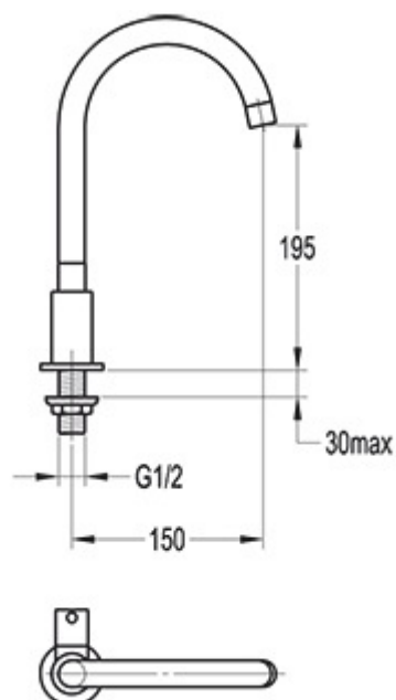
Schéma technique
